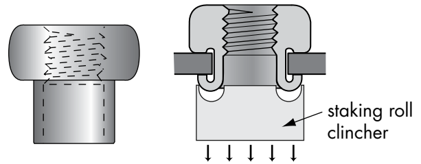
Perma-Nut Insert
