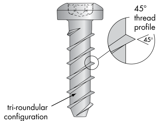
Plastite® 45 Fastener
