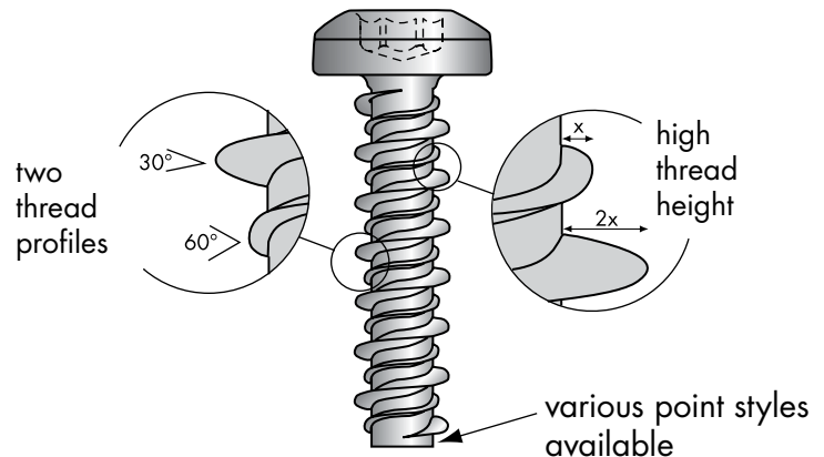
DST Fastener
